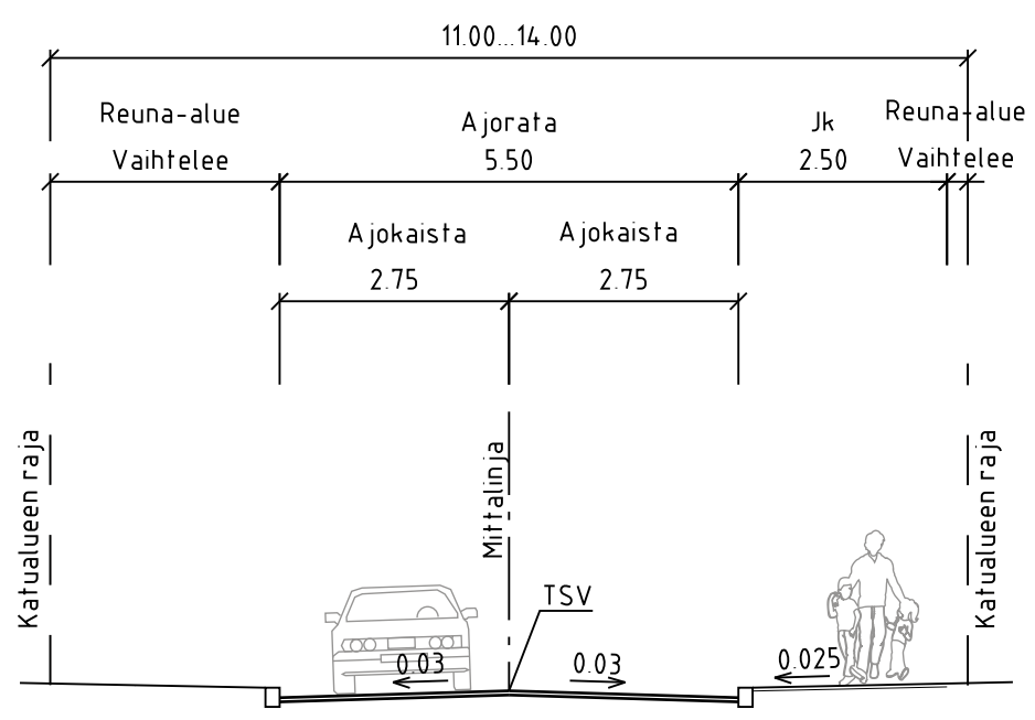
TYYPPIPOIKKILEIKKAUS A-A 1:100
