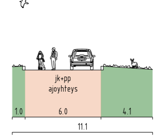
OVIKUJA, LEIKKAUS B - B
