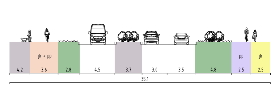
KOIVU-MANKKAANTIE, LEIKKAUS E - E
