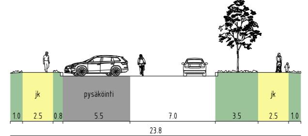
METSÄTONTUNPOLKU, LEIKKAUS D - D
