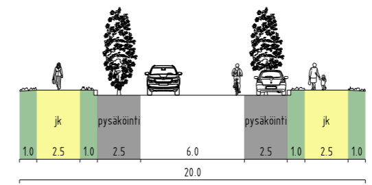
METSÄTONTUNKATU, LEIKKAUS A - A
