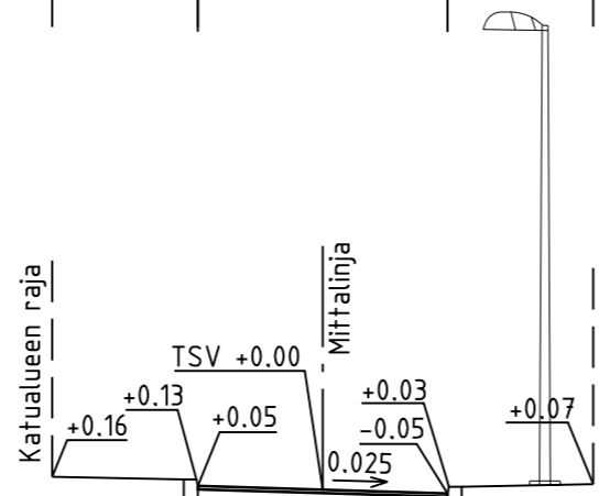
TYYPPIPOIKKILEIKKAUS B-B 1:100
