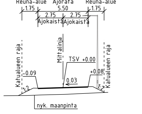
TYYPPIPOIKKILEIKKAUS A-A 1:200
