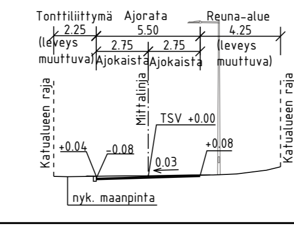
TYYPPIPOIKKILEIKKAUS B-B 1:200
