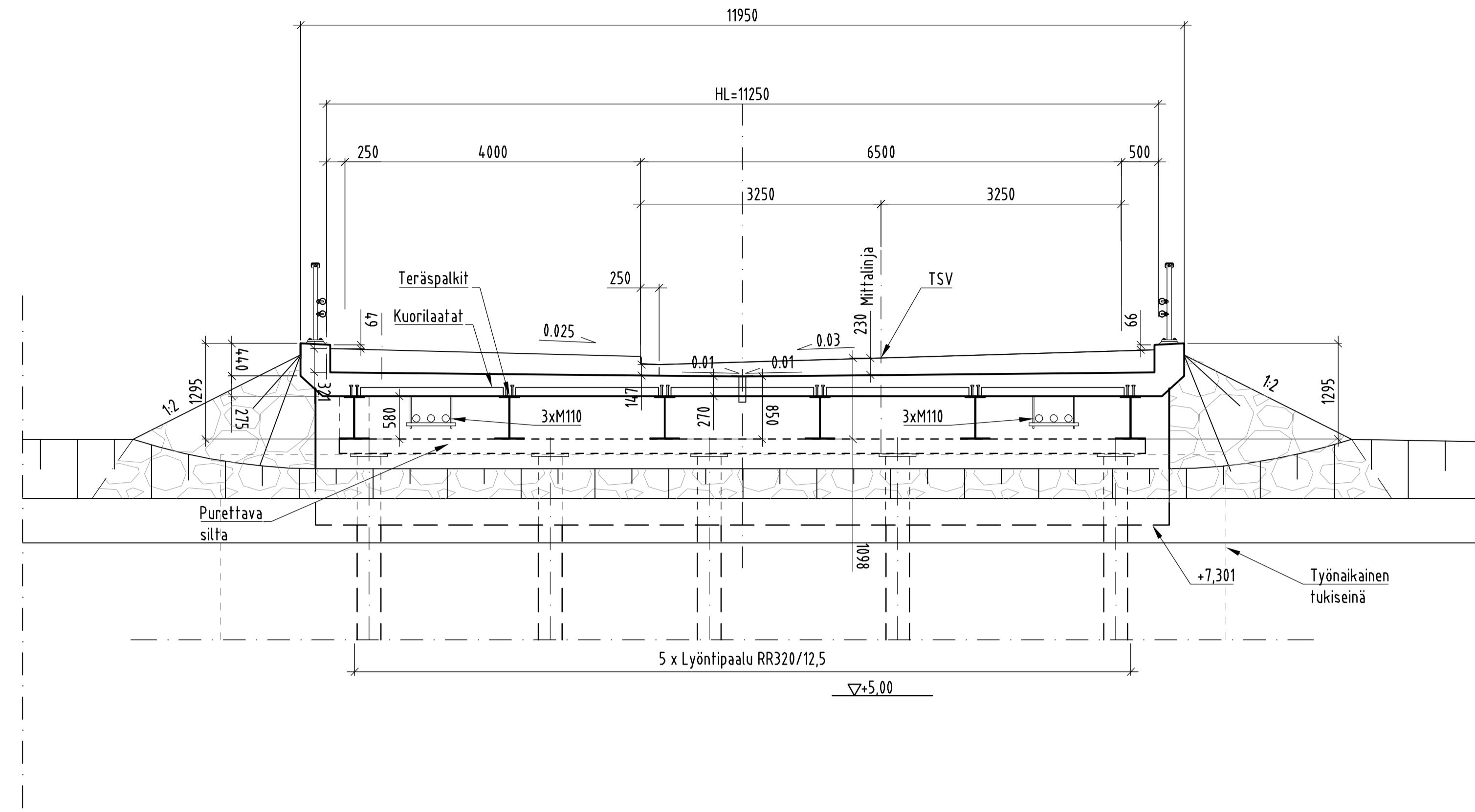
B - B 1:50
