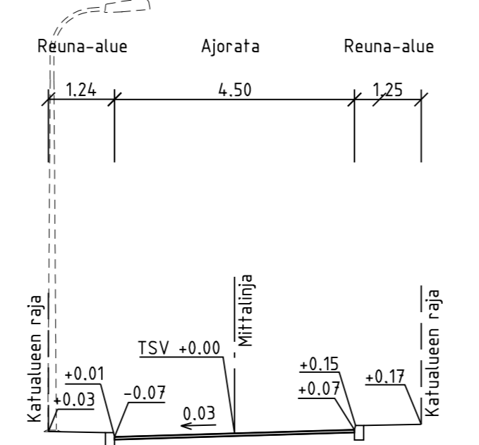
TYYPPIPOIKKILEIKKAUS A-A 1:100
