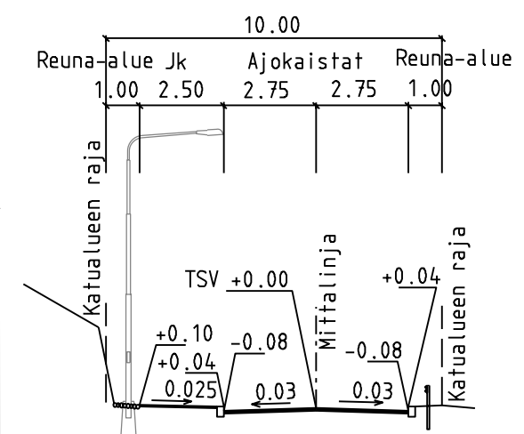
TYYPPIPOIKKILEIKKAUS B-B 1:200
