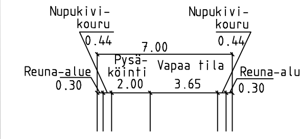
TYYPPIPOIKKILEIKKAUS B-B 1:200
