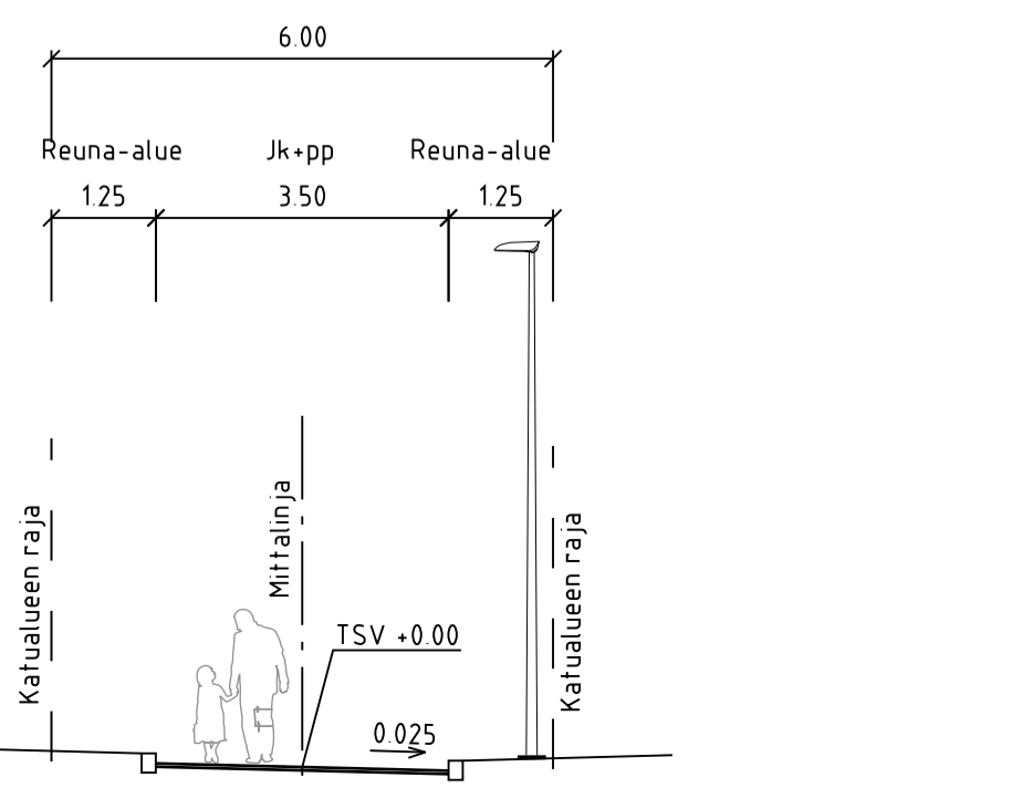
TYYPPIPOIKKILEIKKAUS B-B 1:100
