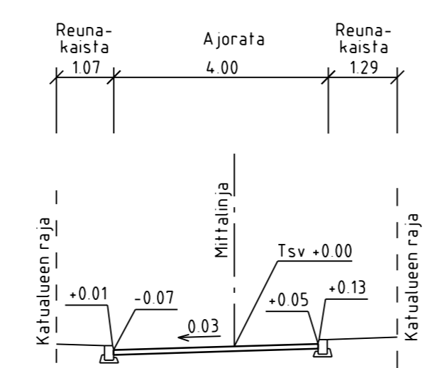
TYYPPIPOIKKILEIKKAUS C-C 1:100
