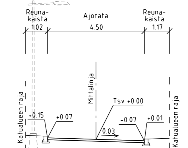
TYYPPIPOIKKILEIKKAUS D-D 1:100
