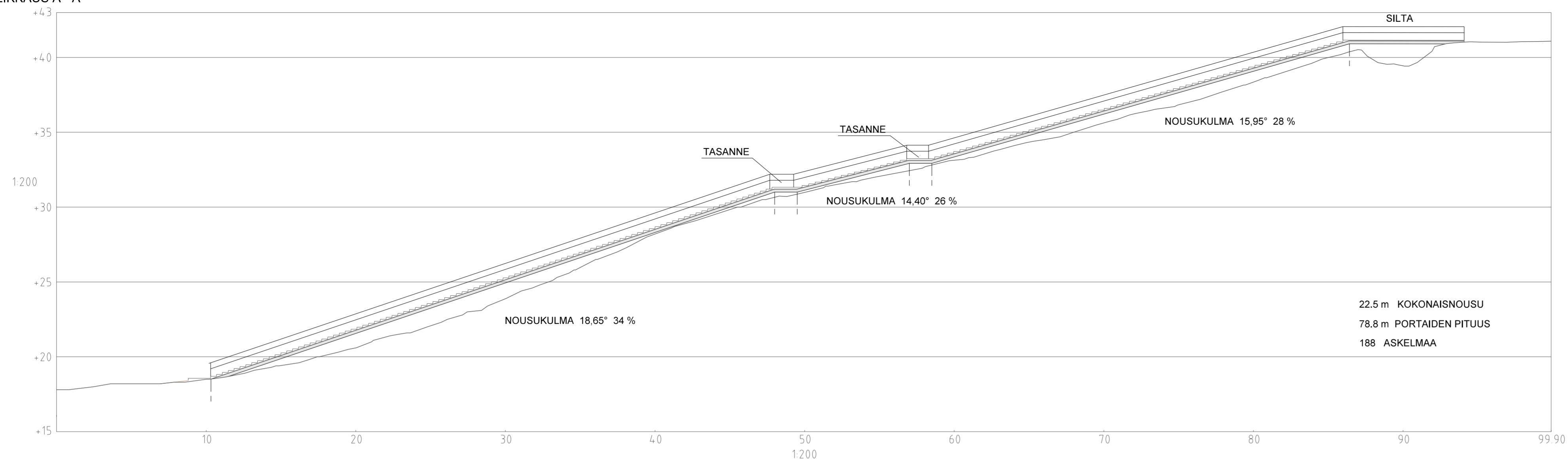
PITUUSLEIKKAUS A - A 1:200
