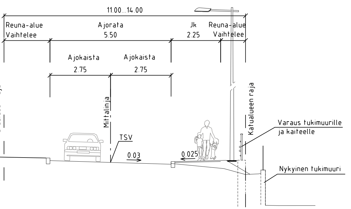
TYYPPIPOIKKILEIKKAUS B-B 1:100
