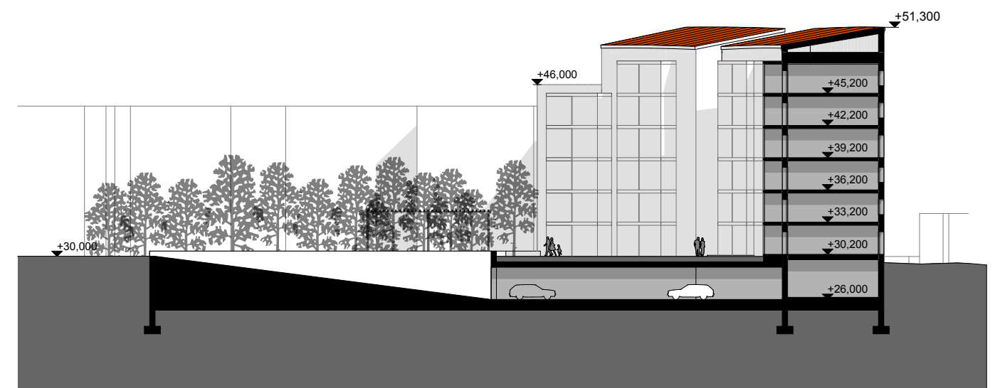
LEIKKAUS Q-Q, S-S & R-R / 1/500
