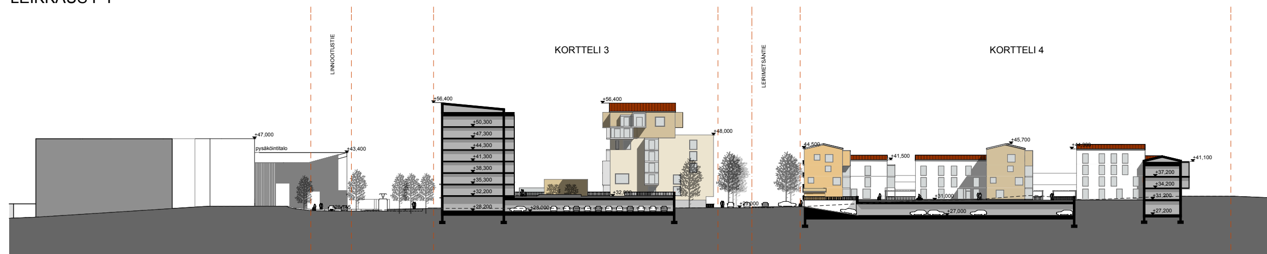
LEIKKAUS F-F
