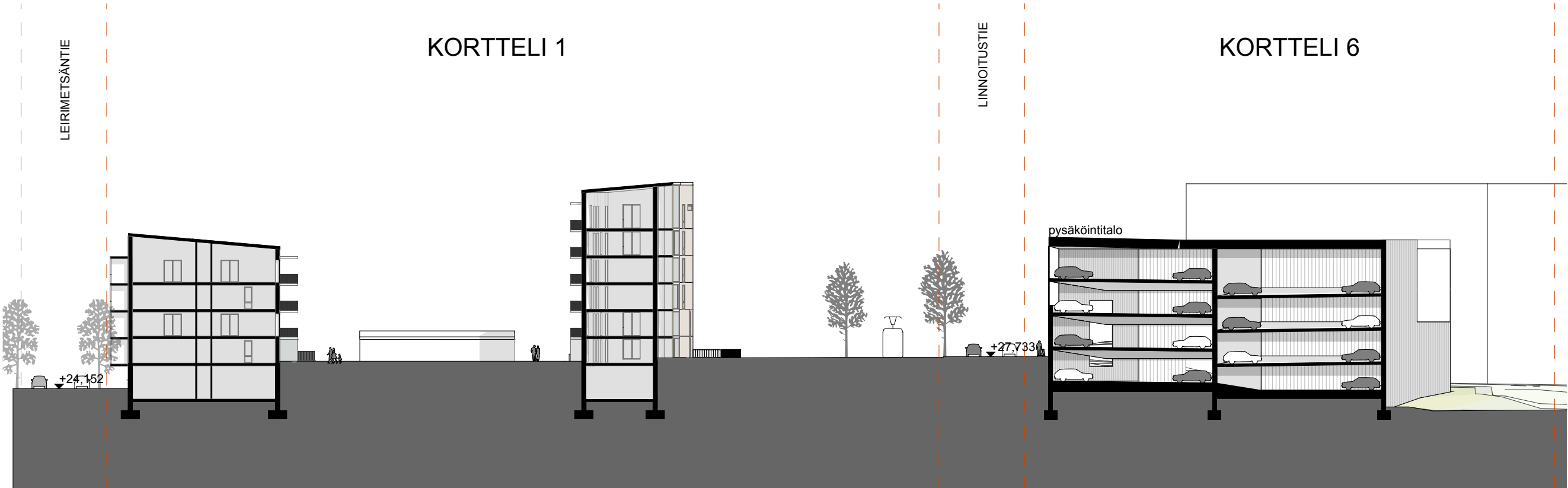
LEIKKAUS P-P & O-O / 1/500
