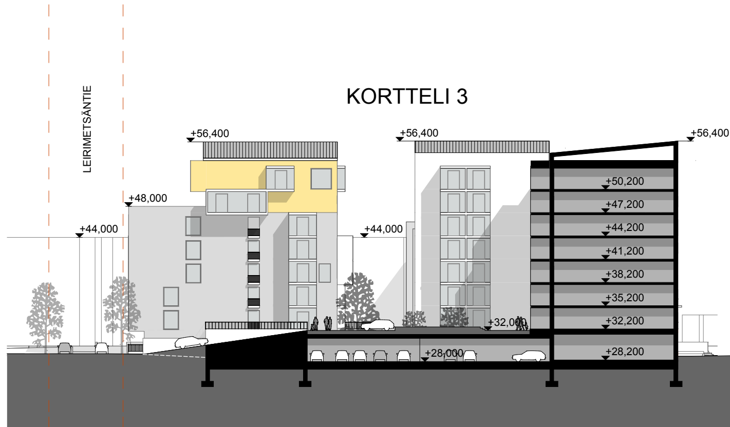
LEIKKAUS Q-Q
