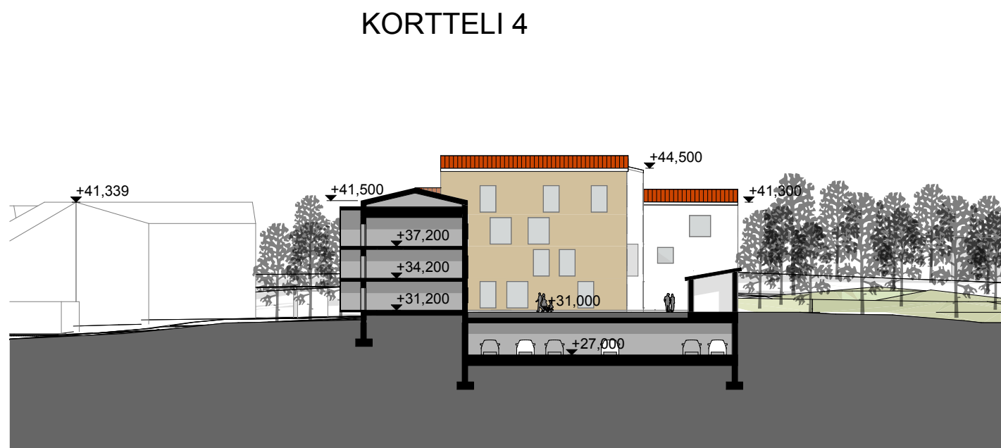
LEIKKAUS Q-Q, S-S & R-R / 1/500
