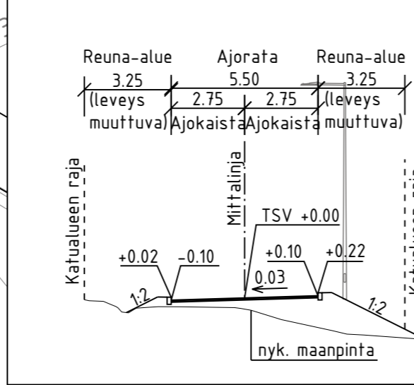
TYYPPIPOIKKILEIKKAUS C-C 1:200
