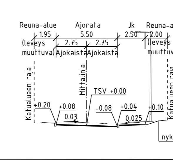
TYYPPIPOIKKILEIKKAUS D-D 1:200
