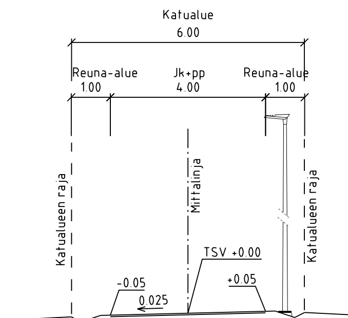
TYYPPIPOIKKILEIKKAUS A-A 1:100
