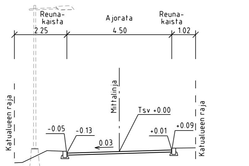
TYYPPIPOIKKILEIKKAUS B-B 1:100
