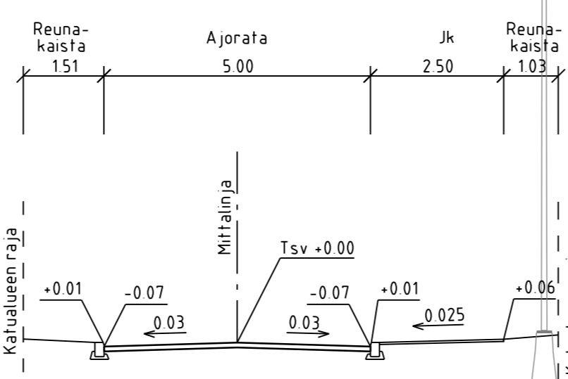
TYYPPIPOIKKILEIKKAUS A-A 1:100
